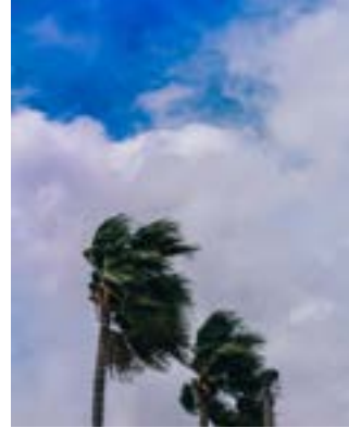
तेज़ हवा
